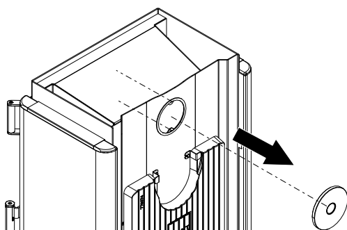
Abb. 24: Abdeckung demontieren
