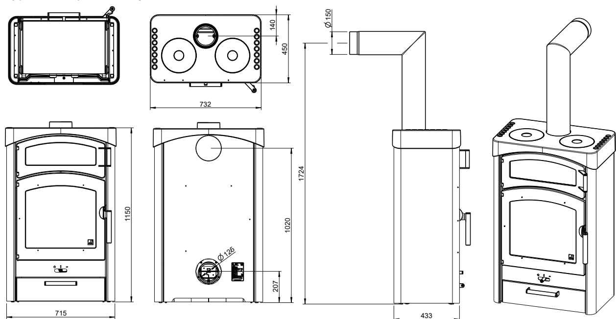
Abb. 1: Abmessungen
