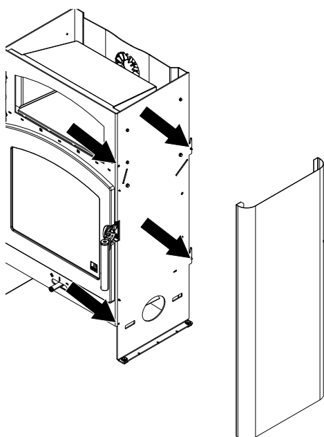
Abb. 10: Seitenverkleidung montieren
