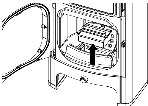
Fig. 56: Rimozione e svuotamento del box cenere
