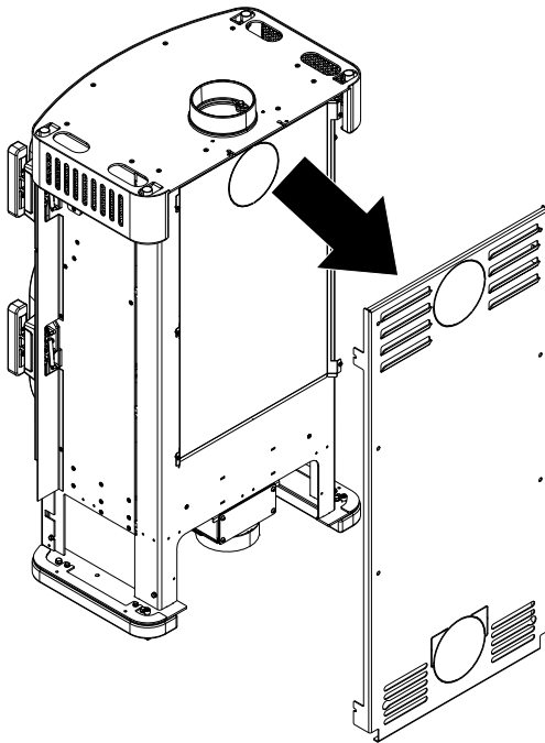
Fig. 61: Rimozione della parete posteriore
