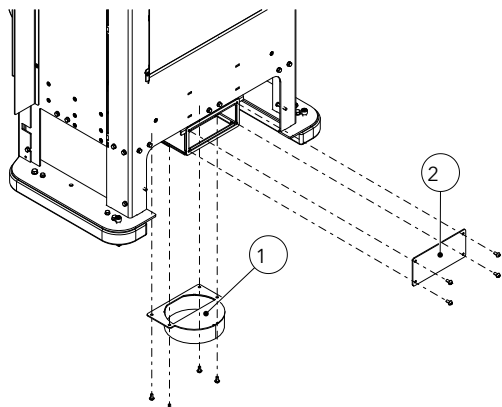
Fig. 38: Smontare la flangia dell'aria di alimentazione
