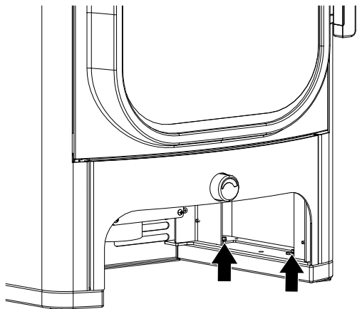
Fig. 22: Svitamento delle viti inferiori
