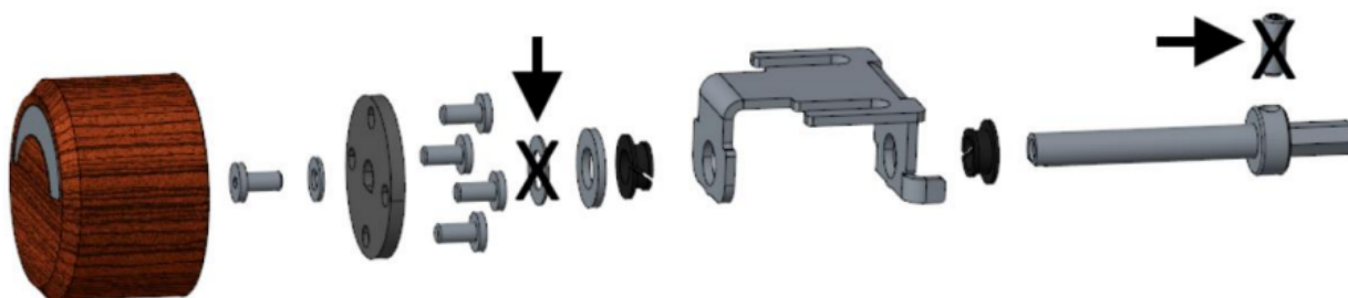
Fig. 43: Modifica dell'unità del controllo rotativo
