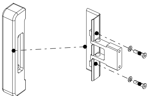
Fig. 26: Montaggio dell'impugnatura in legno
