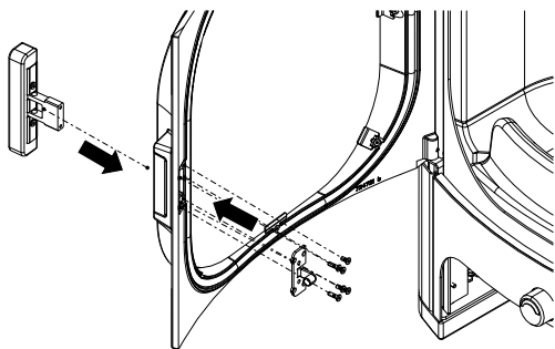
Fig. 27: Montaggio della maniglia nuova
