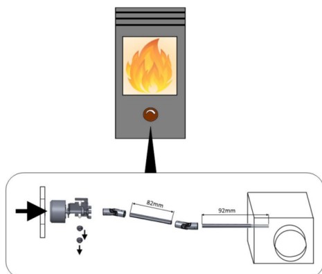
Fig. 41: Rimozione dell'unità del controllo rotativo
