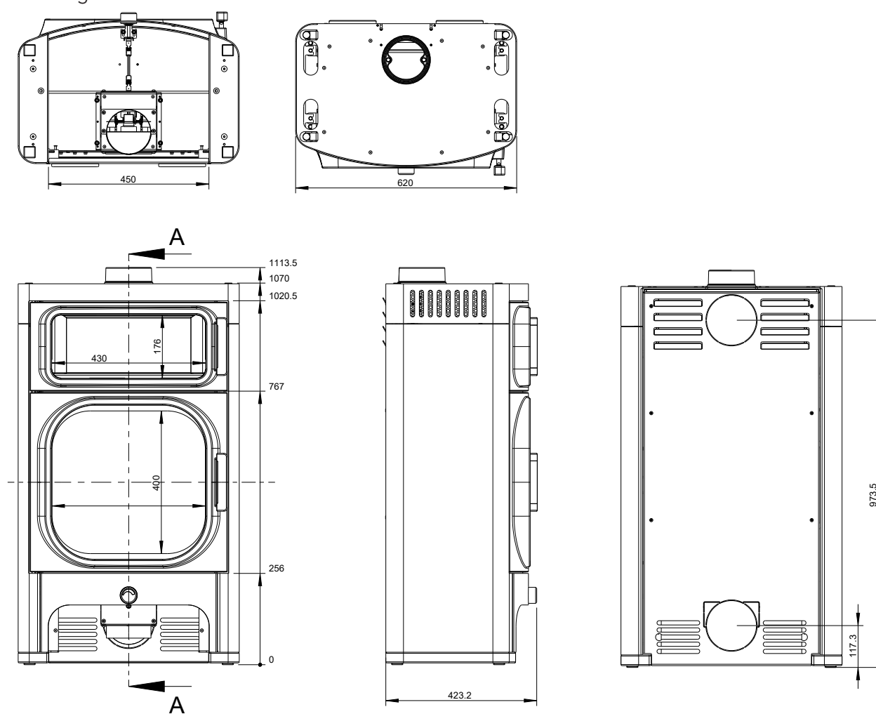
Fig. 1: Dimensioni
