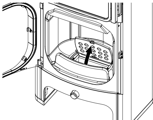
Fig. 53: Sollevamento della griglia
