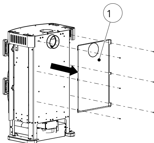
Fig. 32: Smontaggio della protezione anti-irraggiamento
