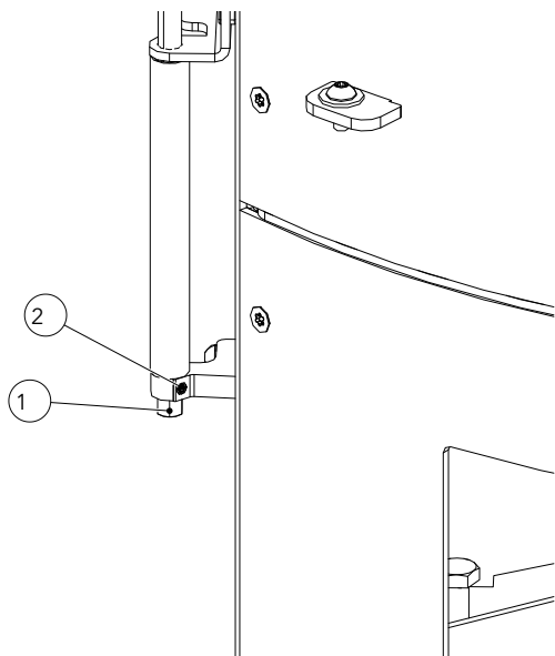
Fig. 48: Regolazione della forza di chiusura dello sportello
