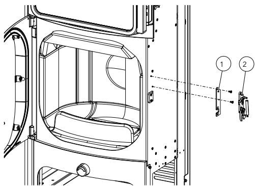
Fig. 28: Montare l'adattatore e il fermo
