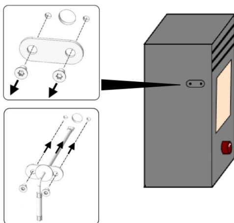
Fig. 42: Fissaggio del sensore di temperatura della camera di combustione
