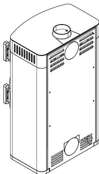
Fig. 36: Montaggio del rivestimento laterale, del coperchio e della piastra di cottura.
