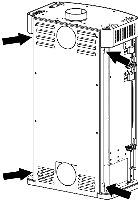
Fig. 60: Svitamento delle viti a sinistra e a destra della parete posteriore.
