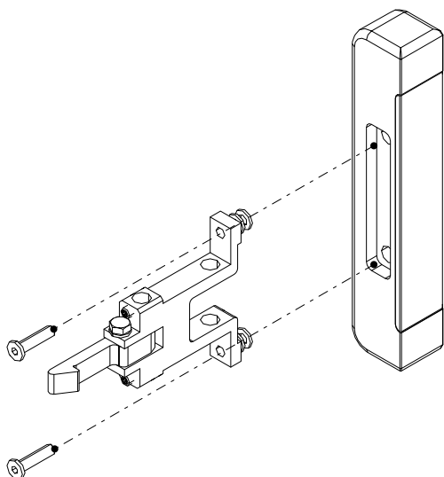
Fig. 25: Rimozione dell'impugnatura in legno
