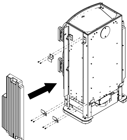
Fig. 34: Montaggio del supporto HMS e della pietra HMS
