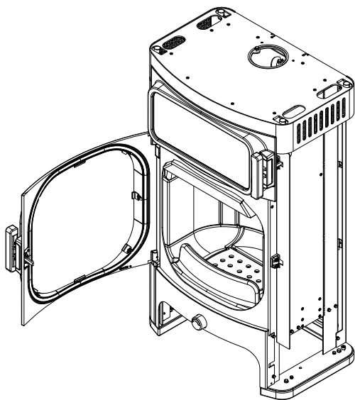
Fig. 24: Apertura dello sportello
