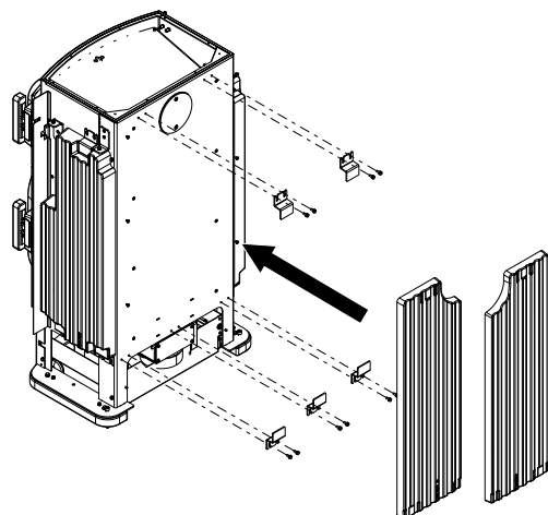
Fig. 35: Montaggio della pietra HMS sul retro
