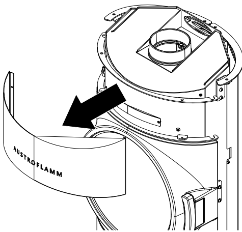
Fig. 13: Rimozione del rivestimento
