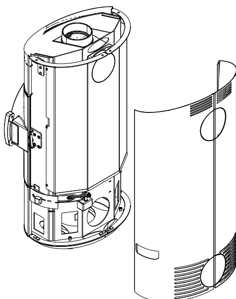
Fig. 10: Rimozione del rivestimento laterale
