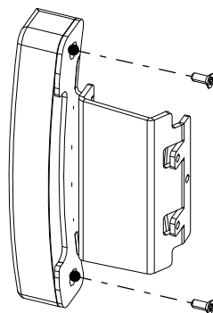
Fig. 21: Montaggio dell'impugnatura in legno
