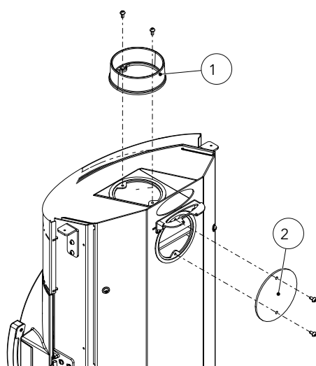
Fig. 30: Smontaggio della presa della canna fumaria e della copertura
