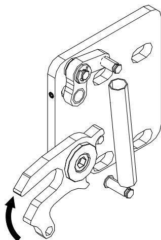
Fig. 24: Incastro del fermo
