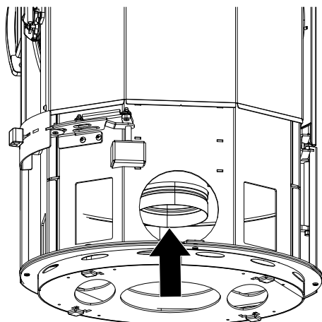
Fig. 35: Fissaggio del tubo Aluflex
