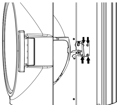
Fig. 26: Regolazione del fermo dello sportello
