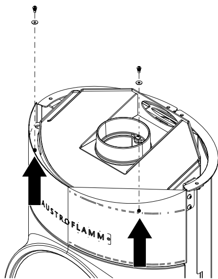
Fig. 38: Svitamento delle viti
