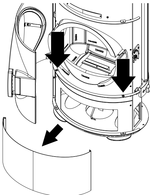
Fig. 43: Smontaggio del rivestimento anteriore
