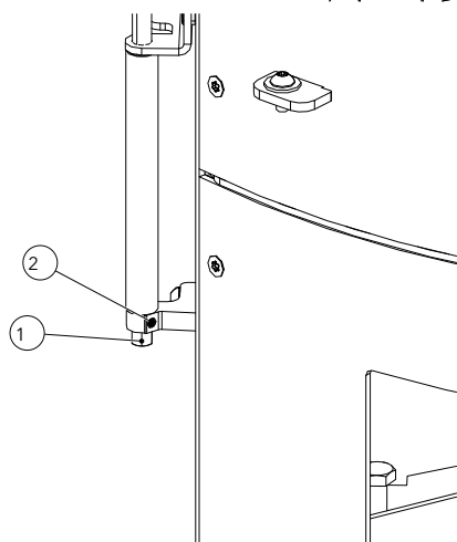
Fig. 44: Regolazione della forza di chiusura dello sportello
