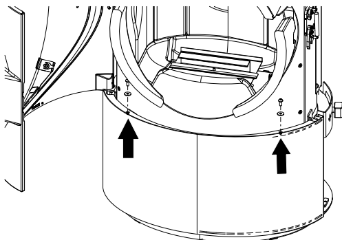
Fig. 14: Svitamento delle viti del rivestimento anteriore inferiore
