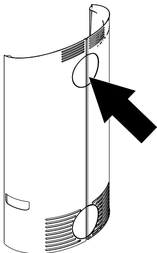
Fig. 28: Rimozione del taglio perforato
