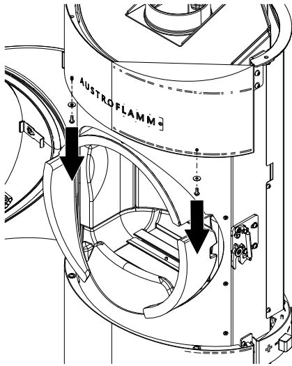
Fig. 12: Svitamento delle viti
