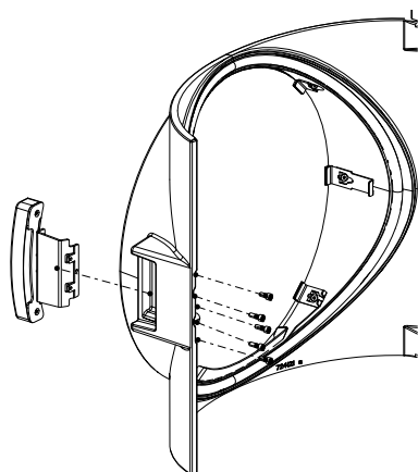
Fig. 22: Montaggio della maniglia della porta
