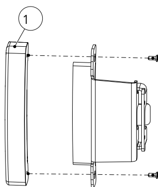
Fig. 20: Rimozione dell'impugnatura in legno
