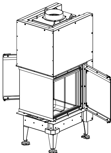
Fig. 73: Déposer le guide d'air secondaire
