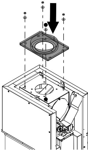
Fig. 24: Installer la plaque d'adaptation
