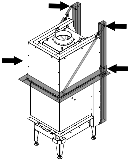
Fig. 44: Installer le cadre porteur sur le châssis de base
