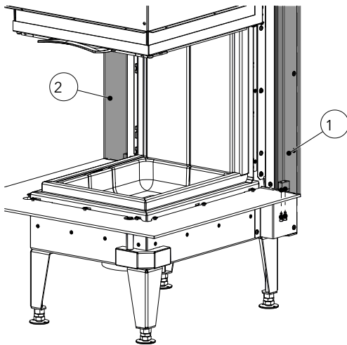
Fig. 37: Fixer le cadre design à gauche/droite
