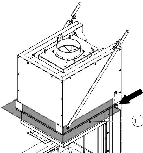
Fig. 38: Fixer le cadre design en haut
