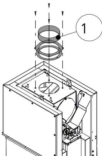
Fig. 23: Démontez la tubulure de fumées
