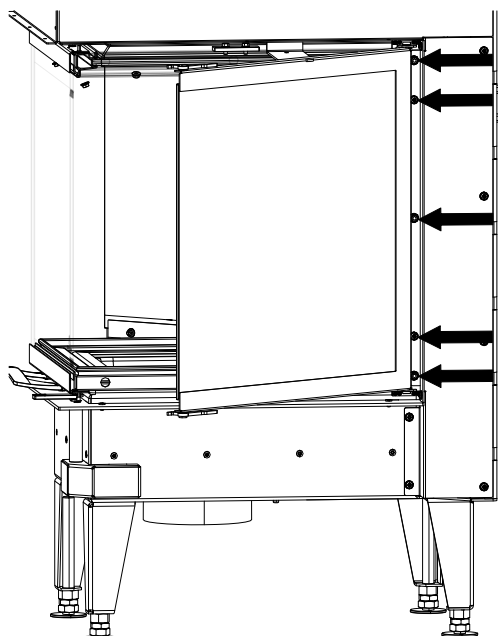
Fig. 77: Déposer la porte
