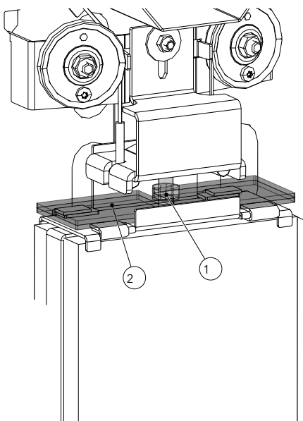
Fig. 64: Mettre en place les poids d'ajustage
