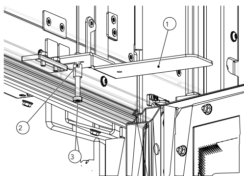
Fig. 76: Dévisser la vis
