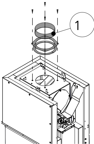
Fig. 25: Démontez la tubulure de fumées
