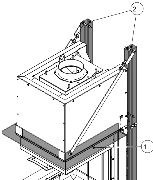
Fig. 39: Installer le cadre design sur le châssis
