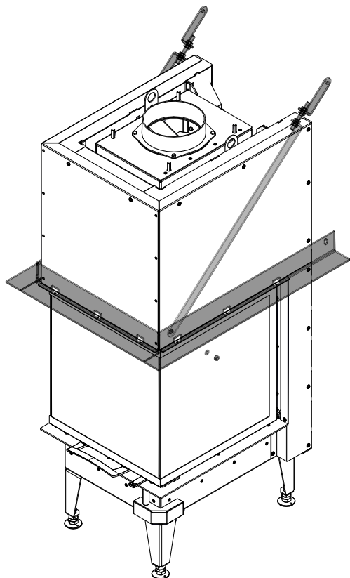
Fig. 43: Fixer et ajuster le cadre porteur
