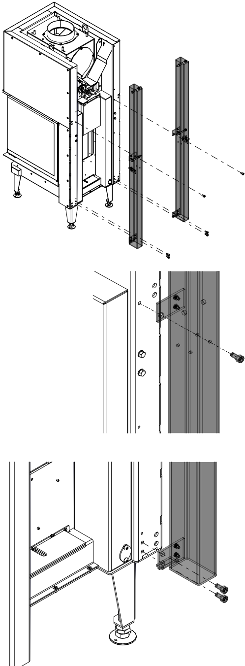
Fig. 46: Installer le châssis de base
