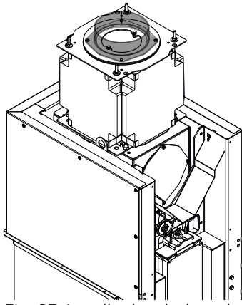
Fig. 27: Installer la tubulure de fumées
