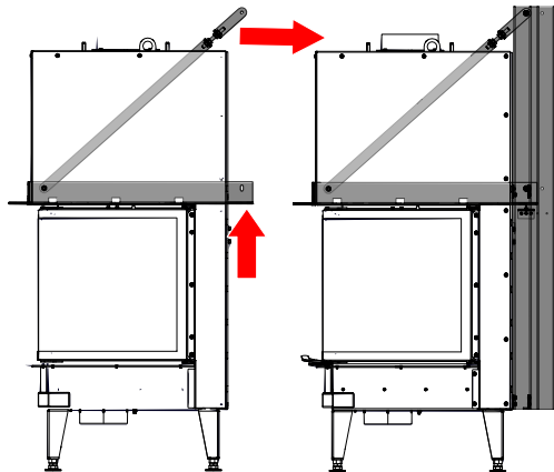
Fig. 45: Ajuster le cadre porteur
