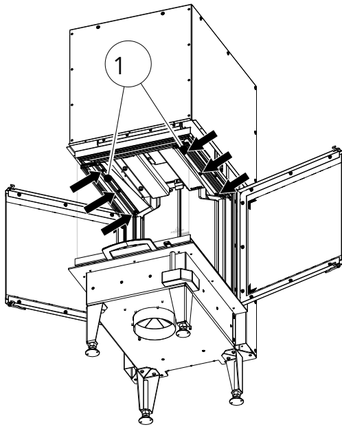
Fig. 74: Enlever les guides d'air secondaire
