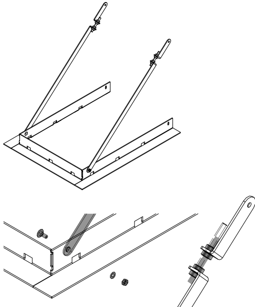
Fig. 35: Assembler le cadre design
