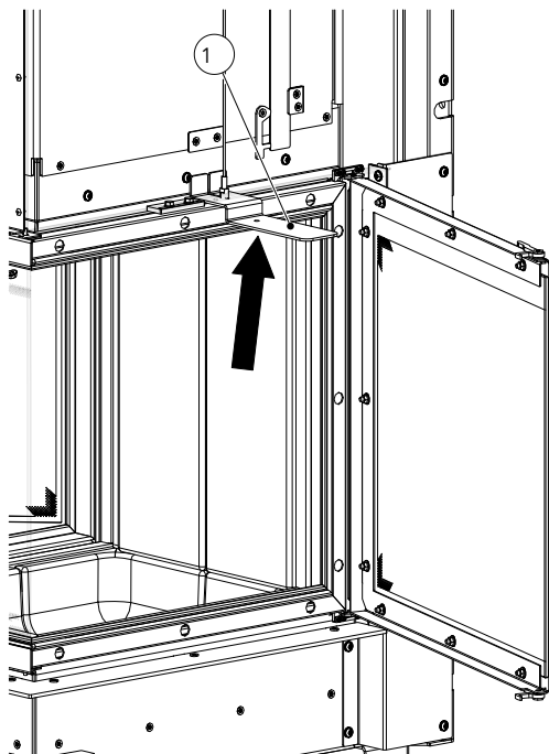
Fig. 75: Poser le serre-câble
