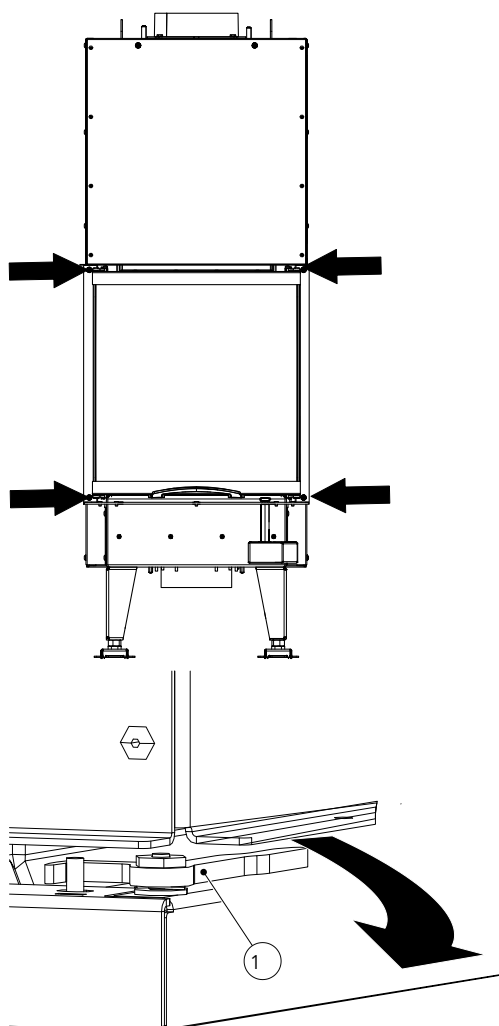
Fig. 72: Ouvrir les crochets de verrouillage
