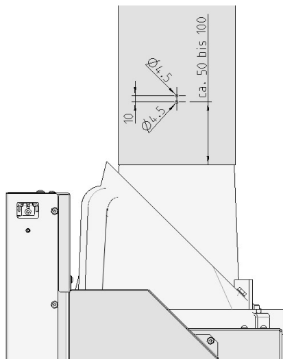
Fig. 49: Schéma de perçage pour conduit de fumée
