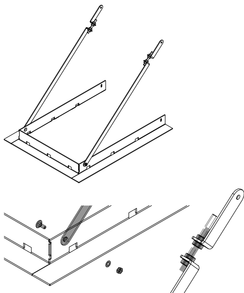
Fig. 42: Assembler le cadre design
