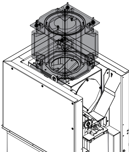
Fig. 26: Installer le caisson d'accumulation
