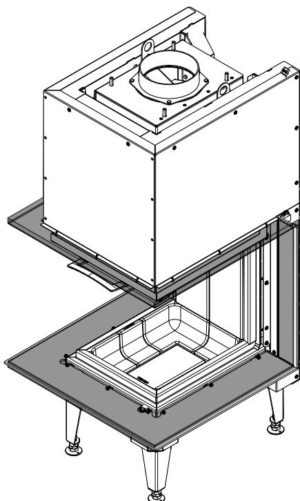
Fig. 32: Installer le cadre design
