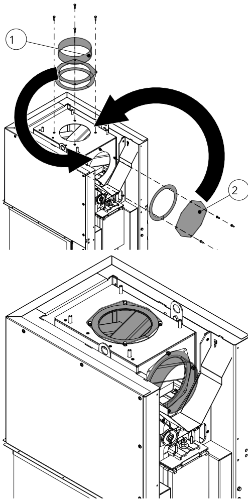
Fig. 22: Modifier le raccordement du conduit de fumée
